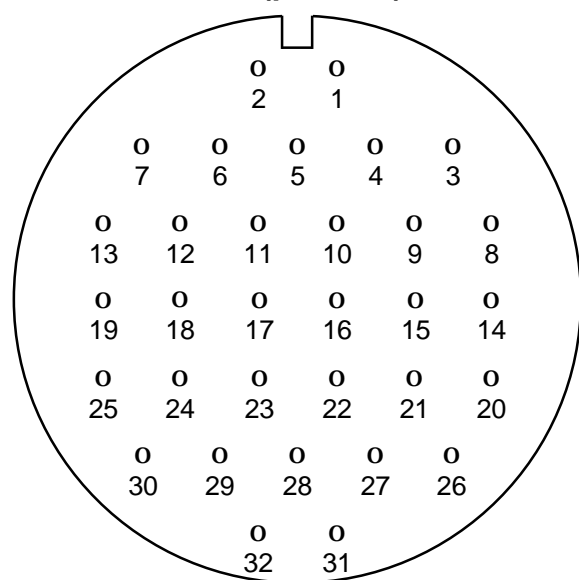
РС 32 (розетка)
