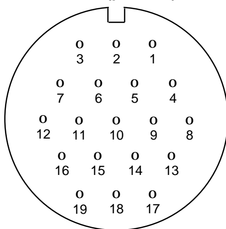
РС 19 (розетка)
